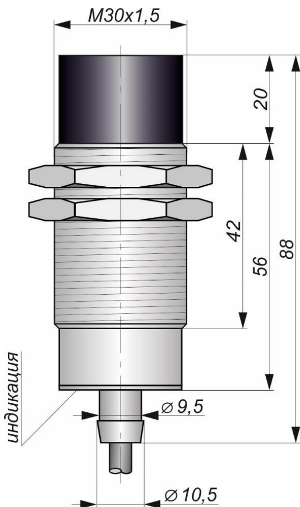
Габаритный чертеж
